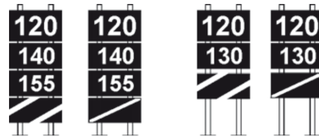
Segnalamento di preavviso
