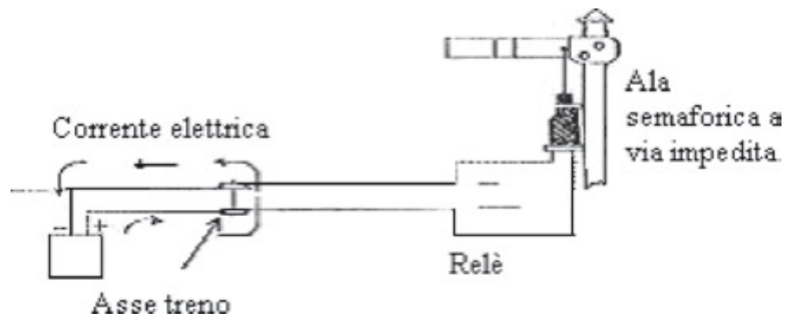
Circuito di binario occupato
