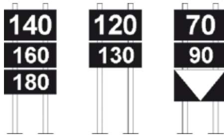
Segnalamento velocità massime
