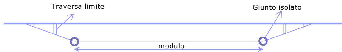
c) In presenza di apparati centrali elettrici e senza tronchini di sicurezza
