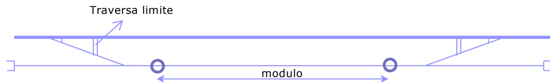
d) In presenza di apparati centrali elettrici e con tronchini di sicurezza
