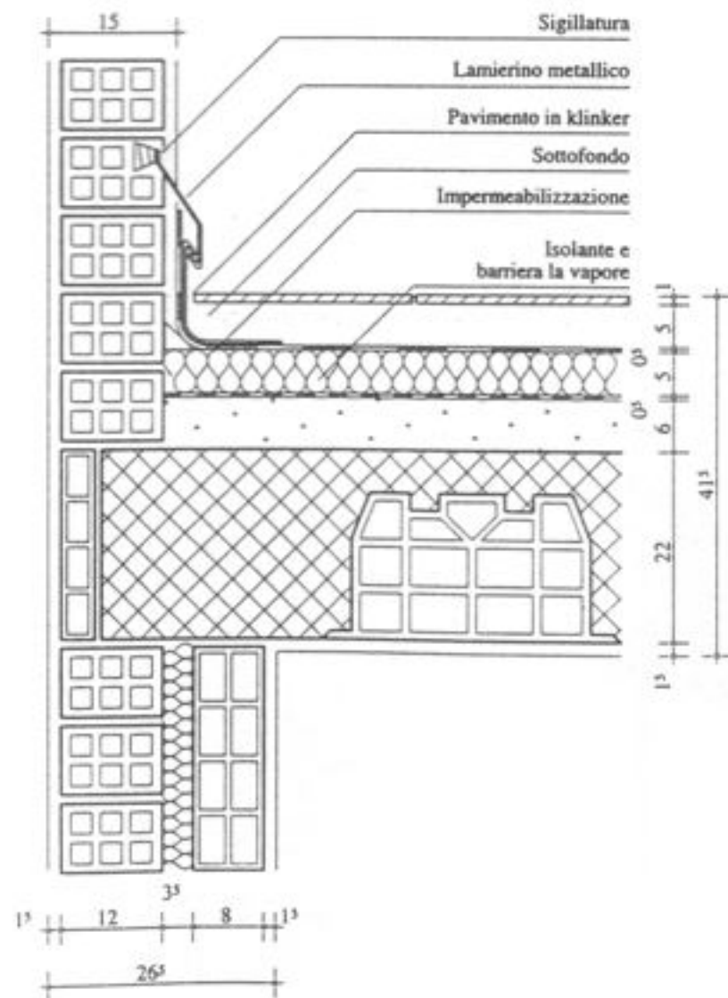
Copertura continua praticabile con manto bituminoso (BPP), pannelli termoisolanti e protezione in piastrelle di klinker
