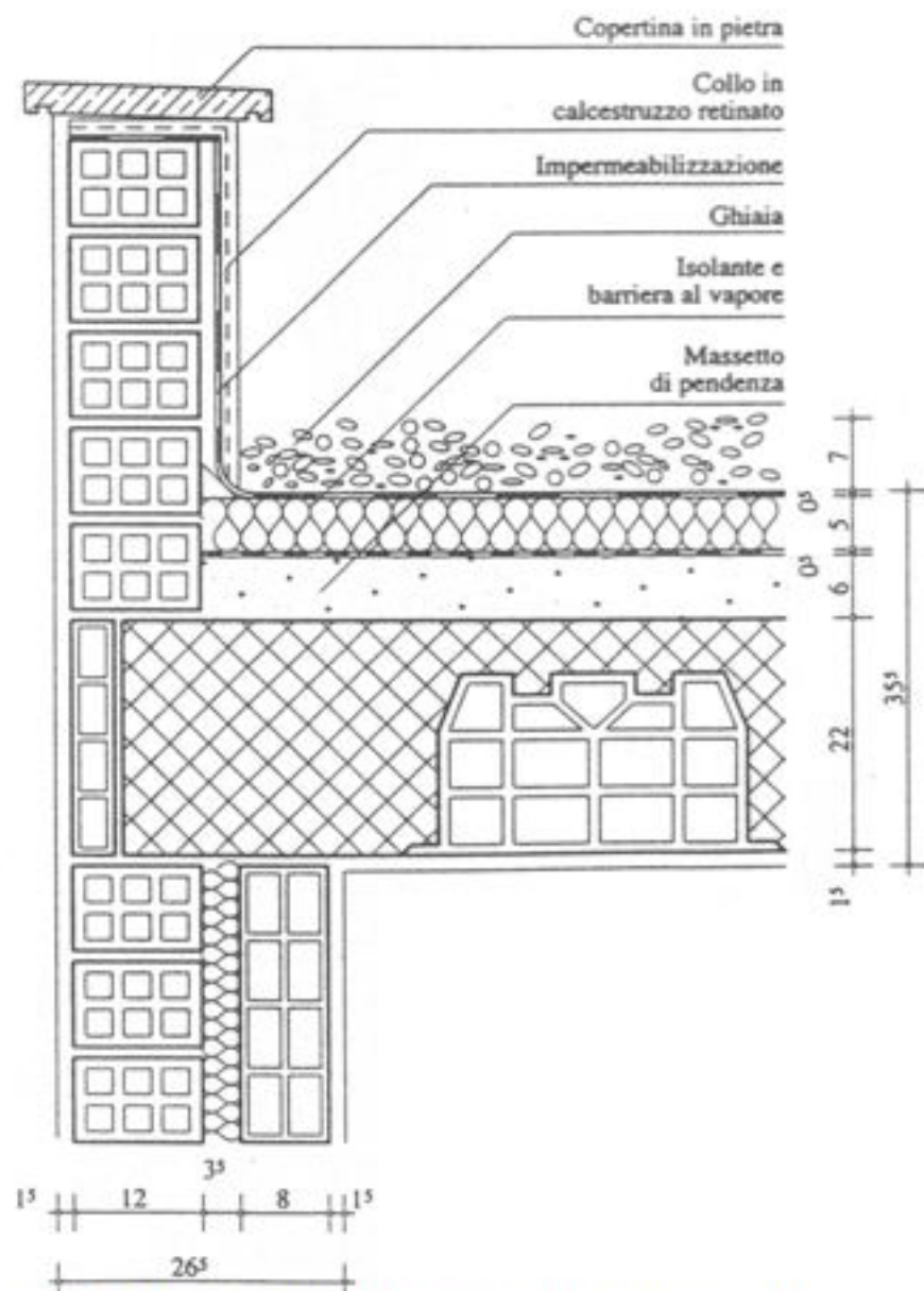
Copertura continua non praticabile con manto bituminoso autoprotetto (BPP), pannelli in schiuma poliuretanicca e protezione in ghiaia
