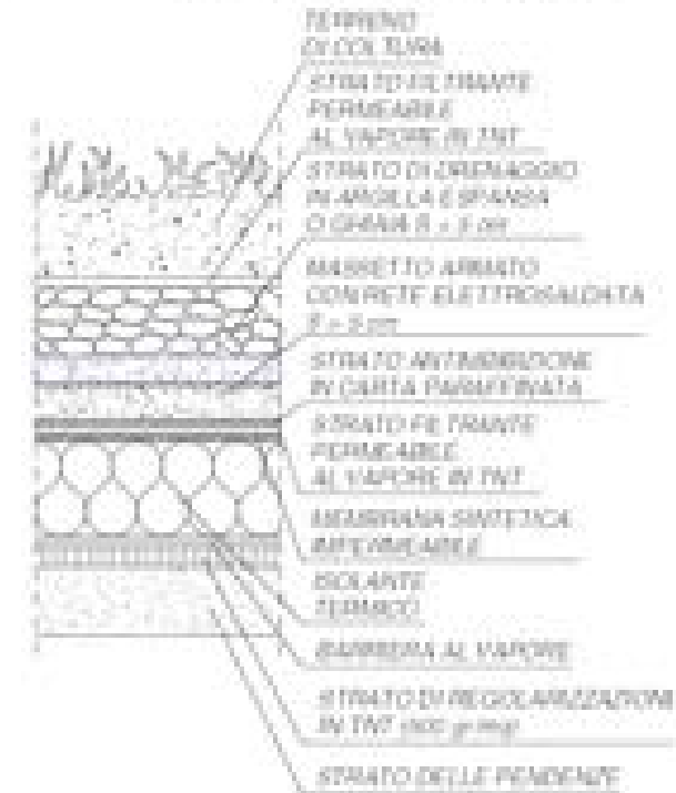
FIG. F.3.5/15 TETTO GIARDINO REALIZZATO CON IL SISTEMA DEL TETTO CALDO
