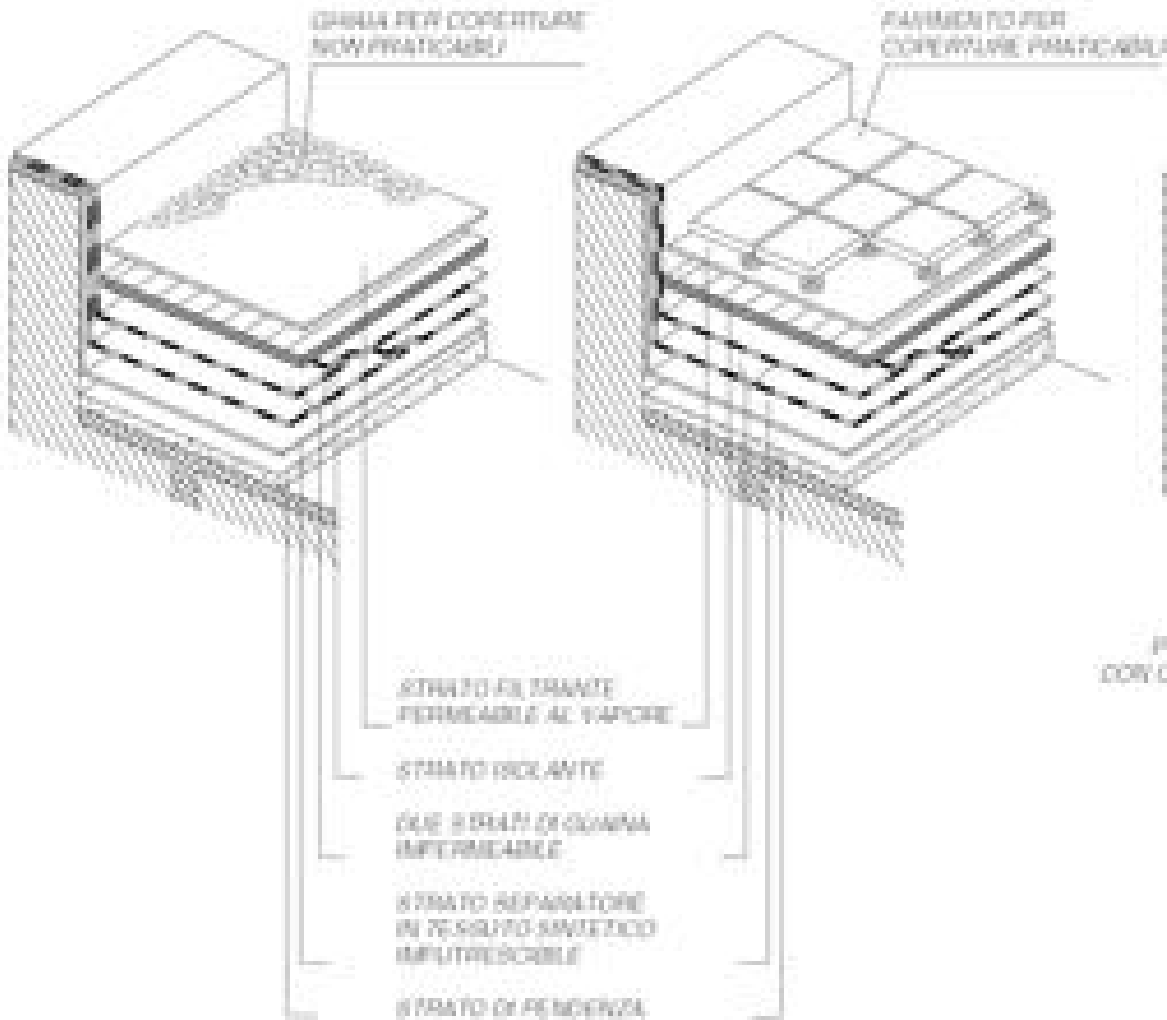
FIG. F.2.1/4 TETTO ROVERSO
