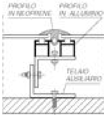
DOBBLIO PROFILO IN ALLUMINIO E NEOPRENE
