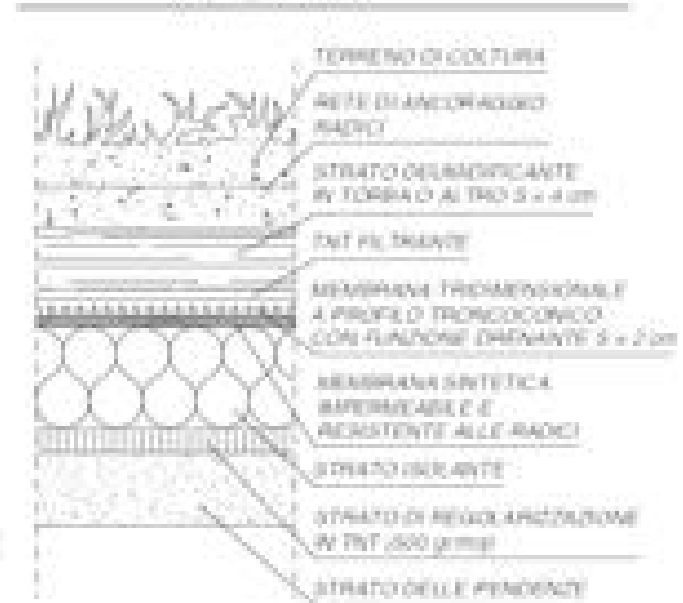
FIG. F.3.5/17 TETTO GIARDINO REALIZZATO CON L'IMPIEGO DI MEMBRANE TRIDIMENSIONALI
