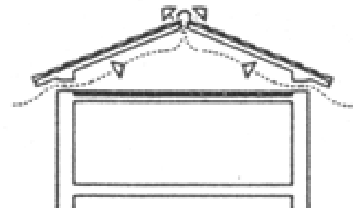
Copertura isolata ventilata
