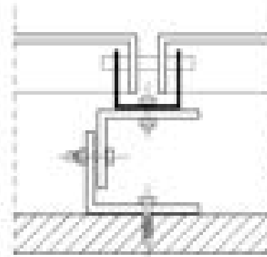
GIUNTO REALIZZATO NEL RIVOLTO LATERALE DEL PANNELLO
