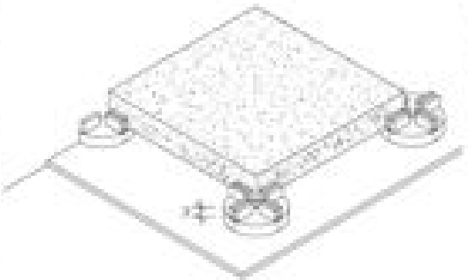
FISSAMENTO SOPRAELEVATO IN QUADROTTI DI CALCESTRUZZO
