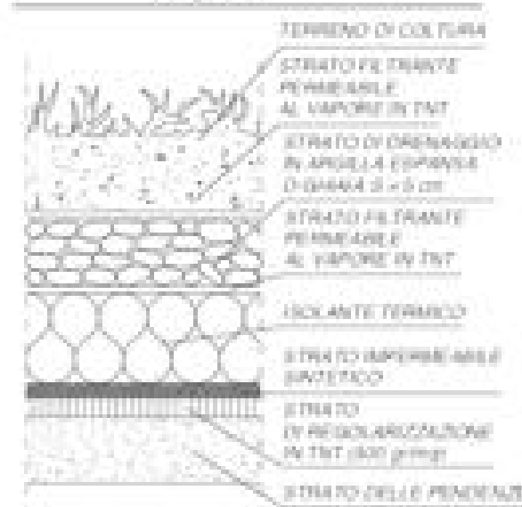
FIG. F.3.5/16 TETTO GIARDINO REALIZZATO CON IL SISTEMA DEL TETTO ROVESCIO
