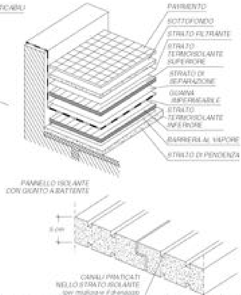
FIG. F.2.1/5 TETTO SANDWICH
