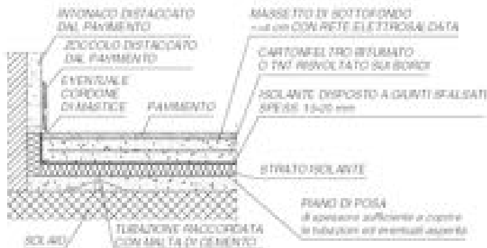
FIG. F.2.3/4 PAVIMENTO GALLEGGIANTE DETTAGLI COSTRUTTIVI
