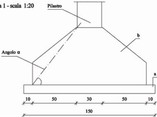
Prospetto frontale tipologia 1 - scala 1:20
