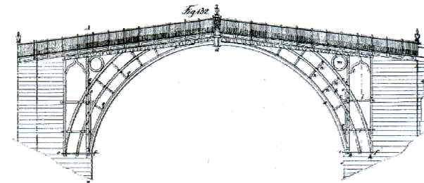
Ponte a Coalbrookdale sul Severn, A Darby, 1775-1779, L=30,6 m ghisa
