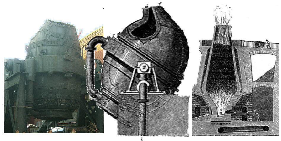
Foto e disegno di un convertitore di Bessemer
