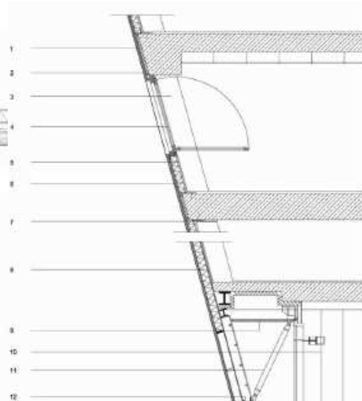
Sezione verticale parete vet - scala 1:50
