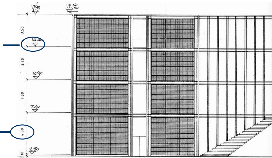
Prospetto Ovest Prospetto laterale Prospetto su Via Rossi
