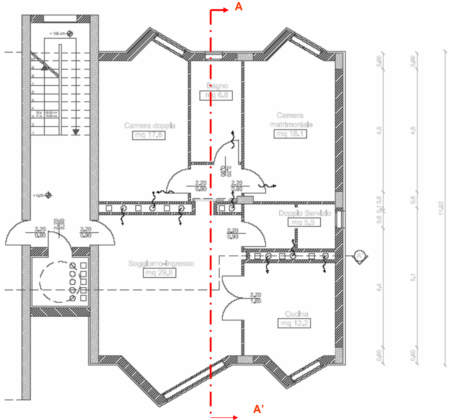
Pianta scala 1:100
